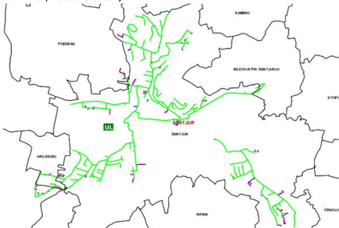
Slika 7: Trasa plinovoda v občini Šentjur
